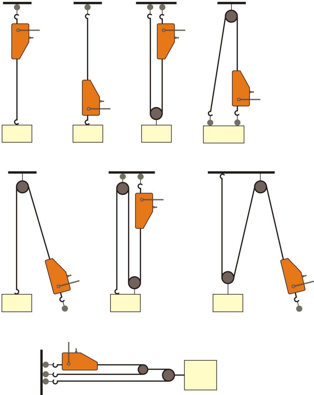
Potenzflaschenzug
